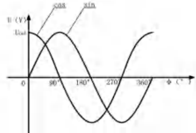
图2输出电压特性 Diagram 2 Output voltage characteristic
