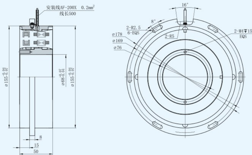
外形及安装尺寸图 Outline(dimension:mm)
