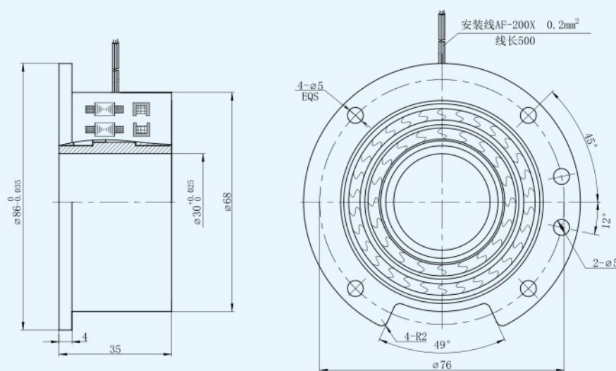
外形及安装尺寸图
