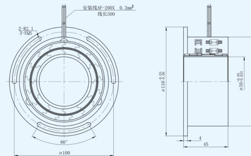
外形及安装尺寸图
