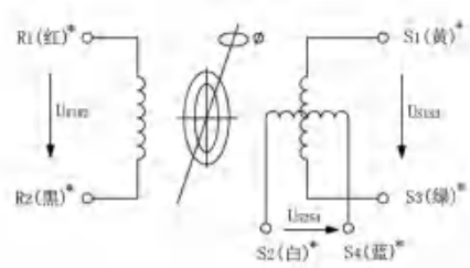
图1接线图 Diagram 1 wiring diagram
