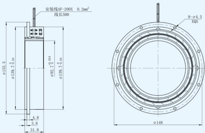
外形及安装尺寸图 Outline(dimension:mm)
